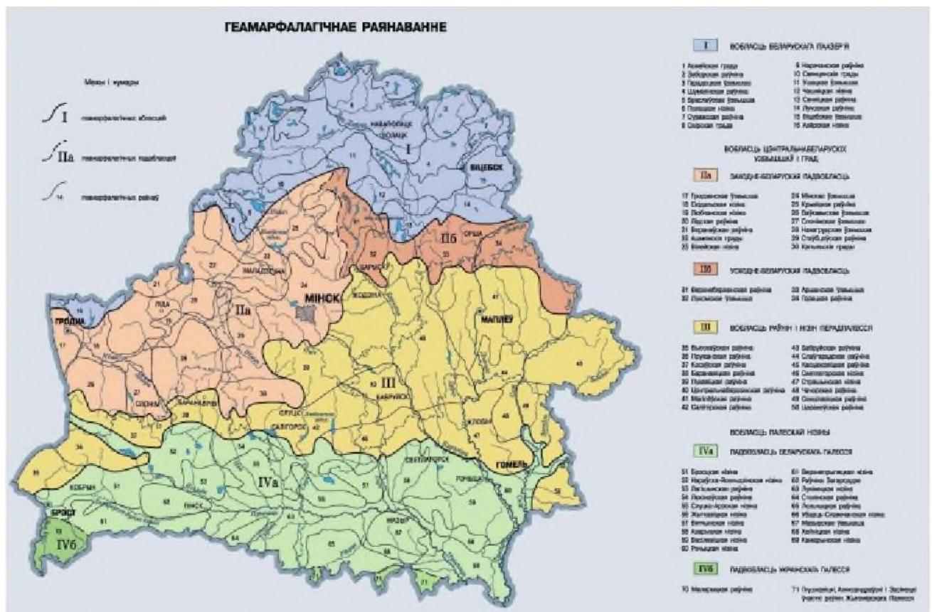
Геоморфологическое районирование РБ
